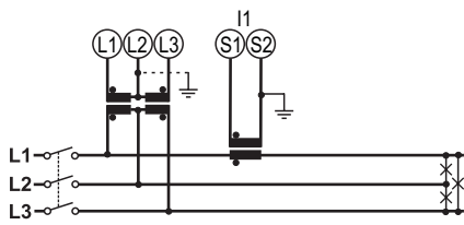
Fig. 14 Sistema trifásico sin neutro (3 hilos), equilibrado, 1 CT y 2 VT/PT.
