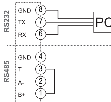
Fig. 25 M C 485232. Puerto serie RS232.
