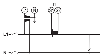
Fig. 18 Sistema monofásico (2 hilos), 1 CT y 1 VT/PT.
